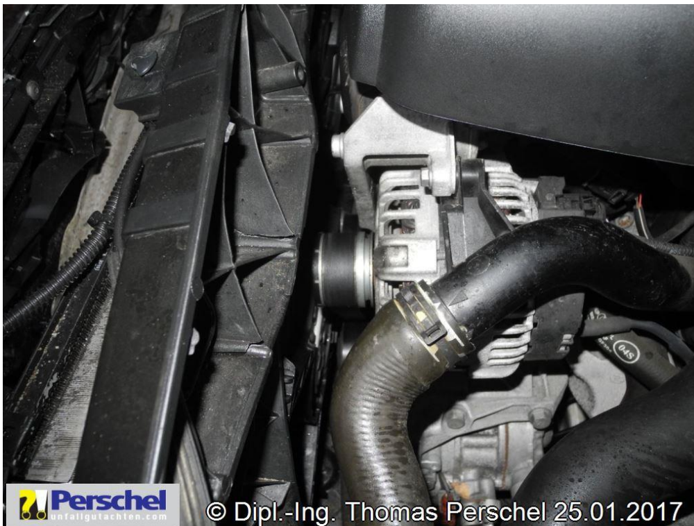
Bild 8: Lüfter beschädigt gegen Motorblock gedrückt
