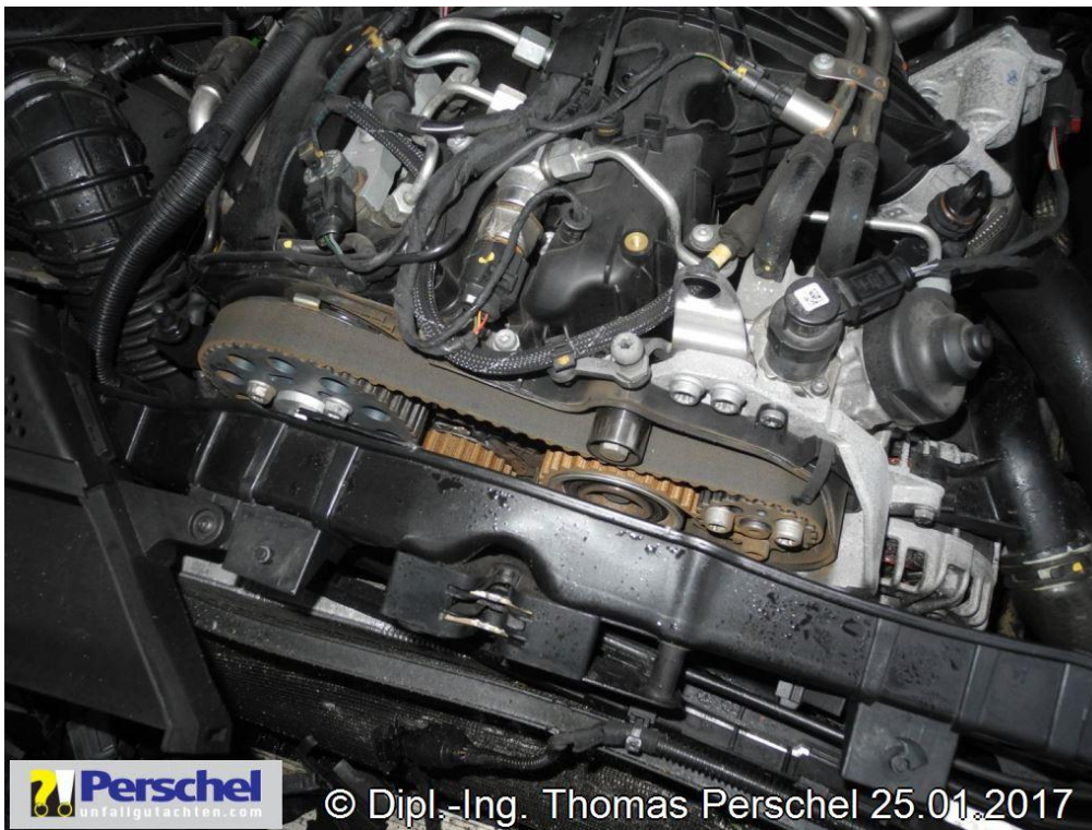
Bild 12: Anstoß gegen Steuerräder ----> Zahnriemen evtl. übersprungen ??
